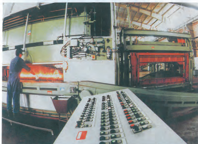
Teilautomatische Biege- und Härtemaschine Semiautomatic Bending and Hardening Machine
