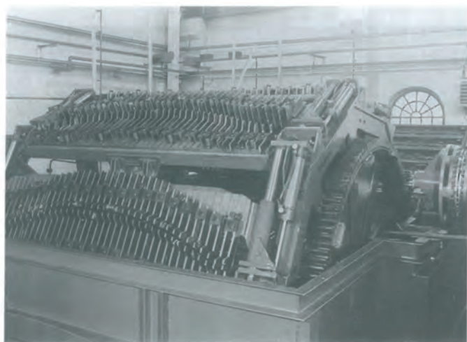
Biege- und Härtemaschine in Trommelausführung Bending and Hardening Machine in Drum Design
