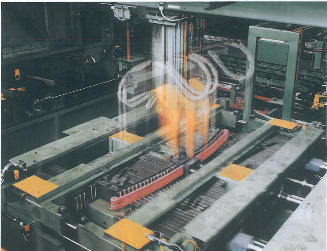
Biege- und Härteanlage (Typ FBH) Bending and Hardening Plant (type FBH)
