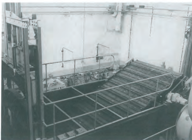
Biege- und Härtemaschine mit 1 Werkzeug Bending and Hardening Machine with 1 Tool
