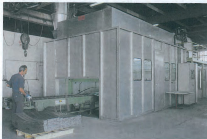
Lackieranlage für Blattfedern Painting Plant for Leaf Springs
