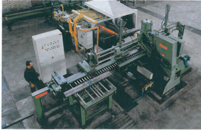
Kombinierte Scher- und Mittenlochanlage Combined Shear- and Center punching plant
